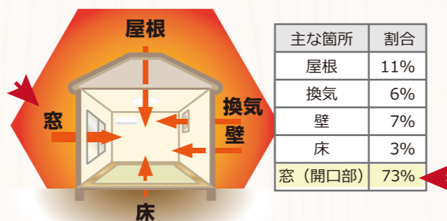
●住まいの外から入ってくる熱の内訳
